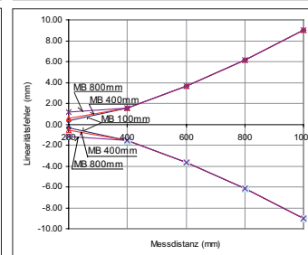
Typische Linearitätsabweichung
