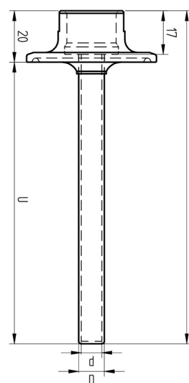
Tri-Clamp Ø 50.5 (BCID: C04) D: Ø10 / Ø12 mm d: Ø8 / Ø10 mm
