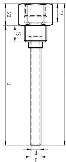
G 1/2 A ISO 228-1 (BCID: G06) D: Ø10 / Ø12 mm d: Ø8 / Ø10 mm
