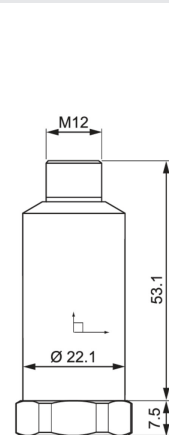
Gehäuse mit Steckverbindung M12-A, 4-Pin
