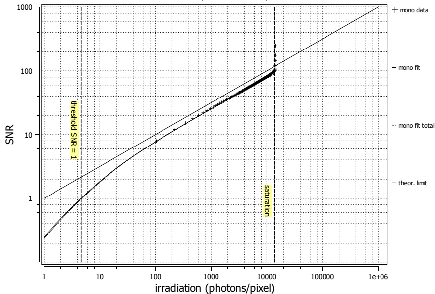
SNR mACC300044, 533 nm, 14.03.2023
