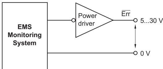
Blockschaltbild/Block diagram
