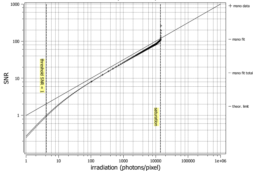
SNR mACC300034, 533 nm, 09.03.2023
