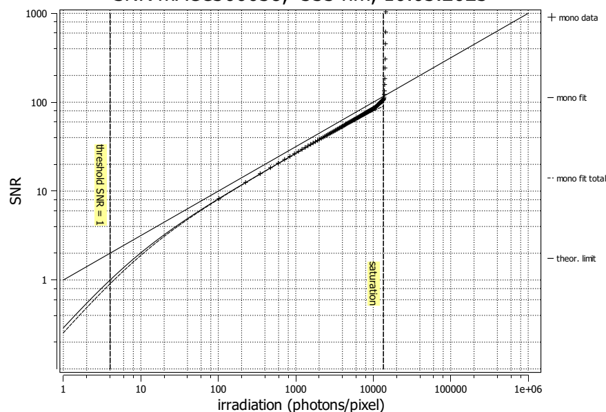
SNR mACC300038, 533 nm, 10.03.2023
