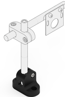
Montagezeichnung
