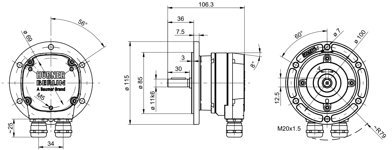
Vollwelle, Kabelverschraubung
