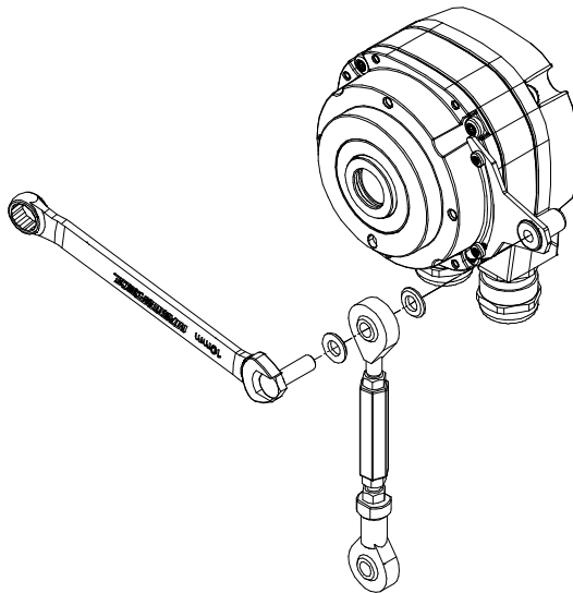
Abb. 3: Drehmomentstütze demontieren
