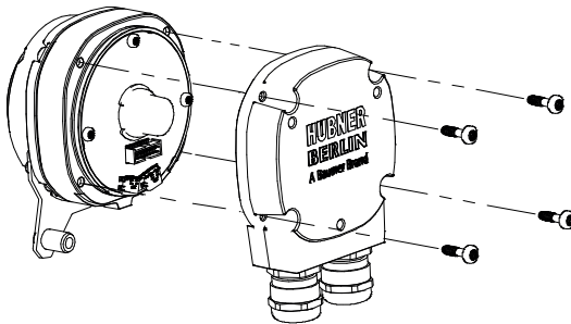
Abb. 13: Klemmenkasten demontieren
