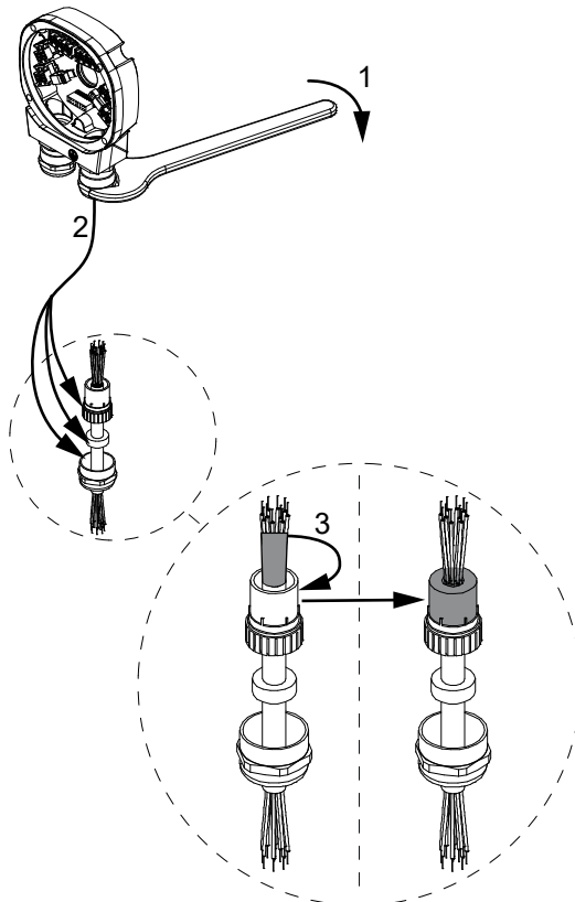
Abb. 7: Kabel vorbereiten
