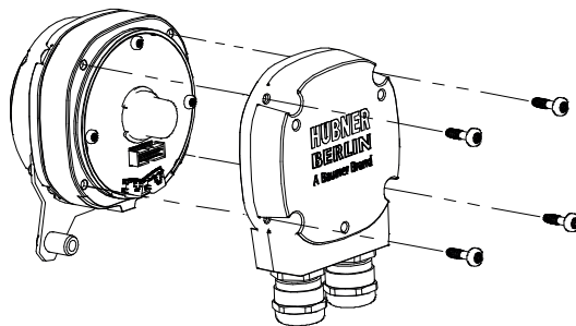
Abb. 12: Klemmenkasten montieren
