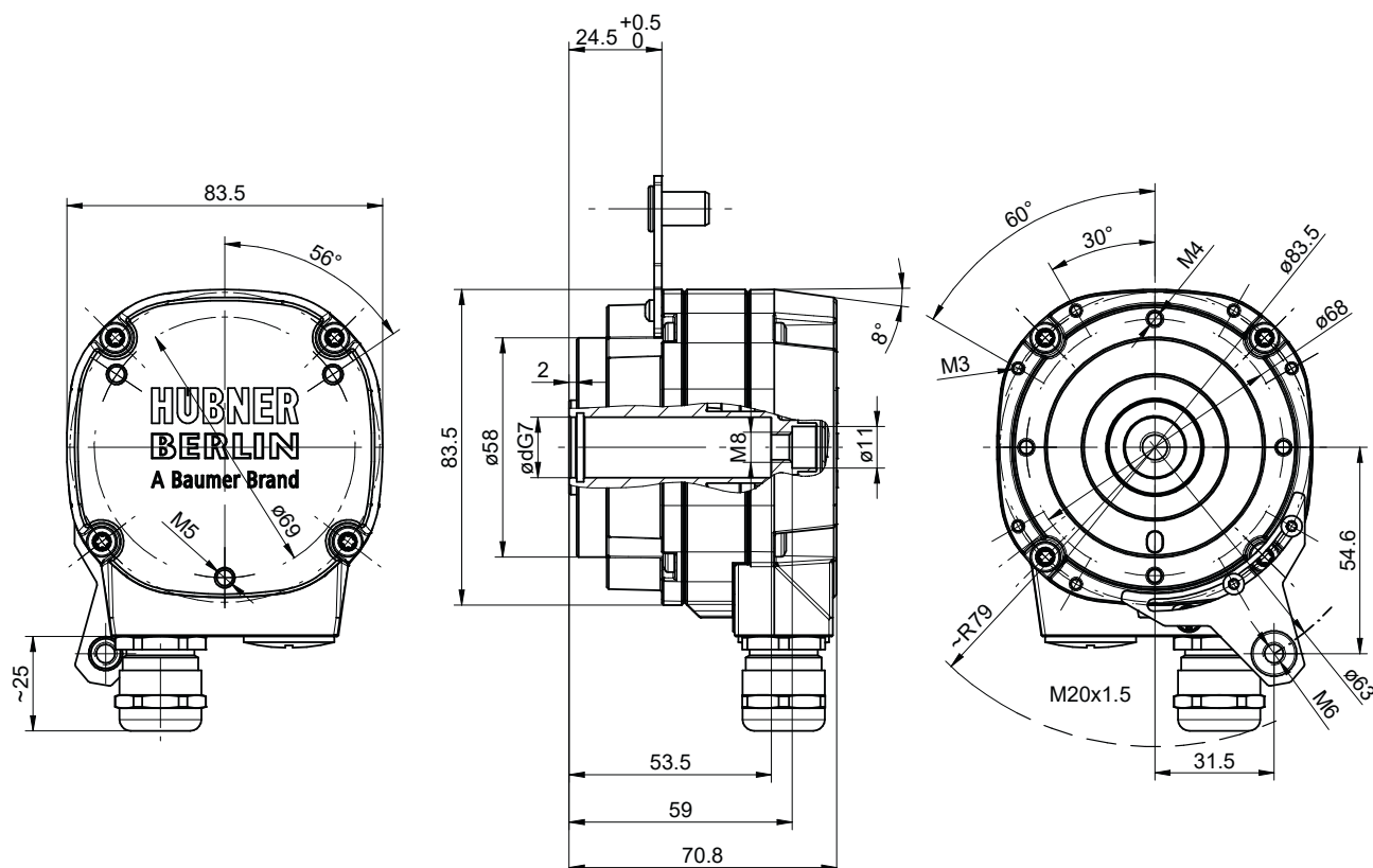
Abb. 16: Abmessungen der einseitig offenen Hohlwelle (Abmessungen in mm, wenn nicht anders angegeben)
