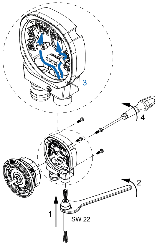
Abb. 8: Kabel anschliessen
