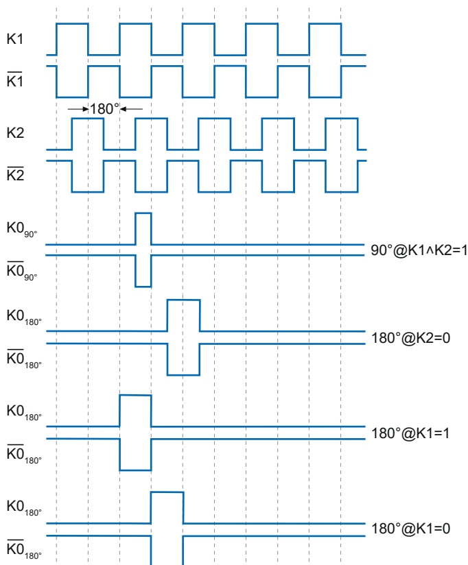
Abb. 10: Ausgangssignale bei positiver Drehrichtung
