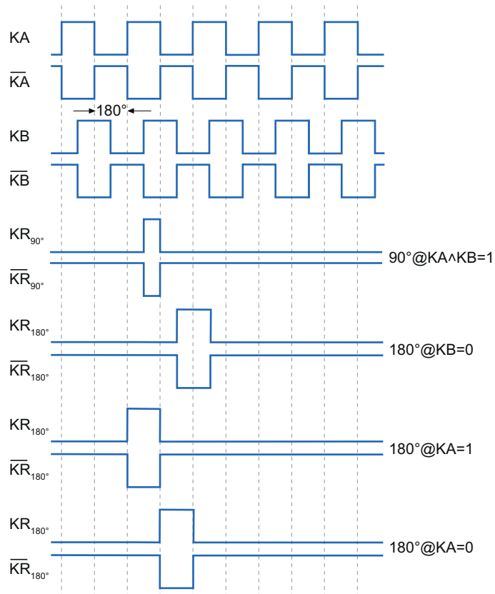
Abb. 11: Ausgangssignale bei positiver Drehrichtung
