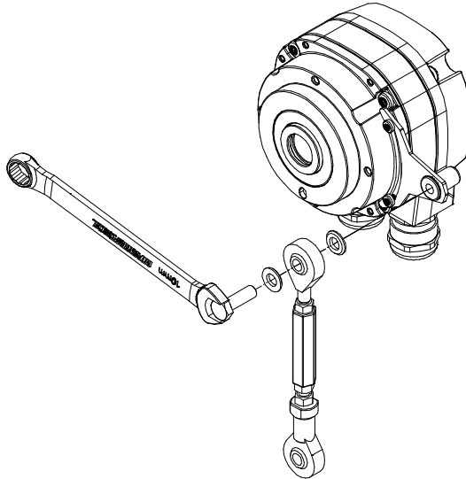
Abb. 14: Drehmomentstütze demontieren
