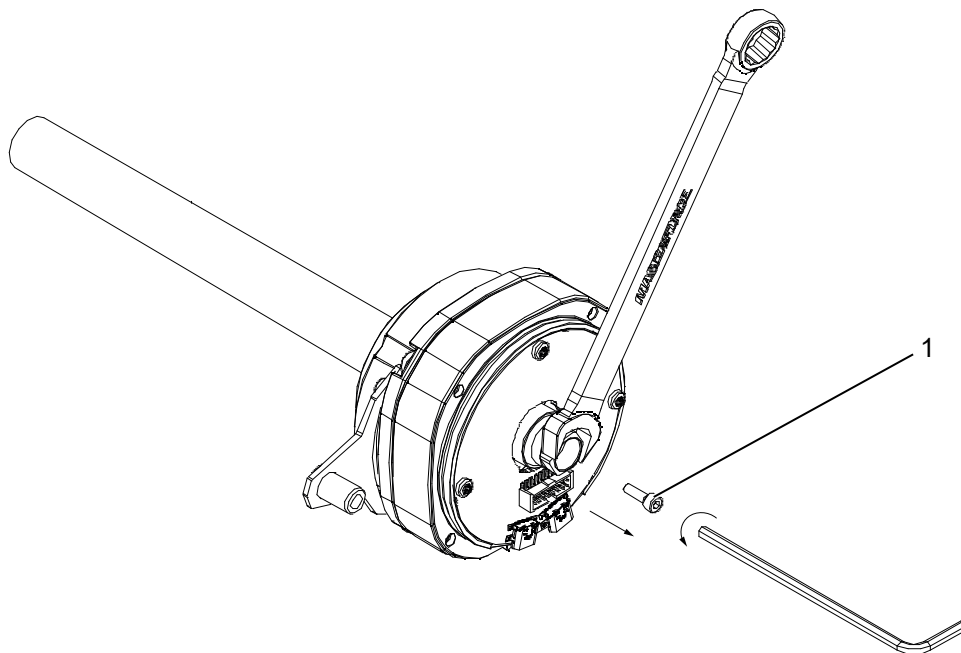
Abb. 15: Zylinderschraube demontieren
