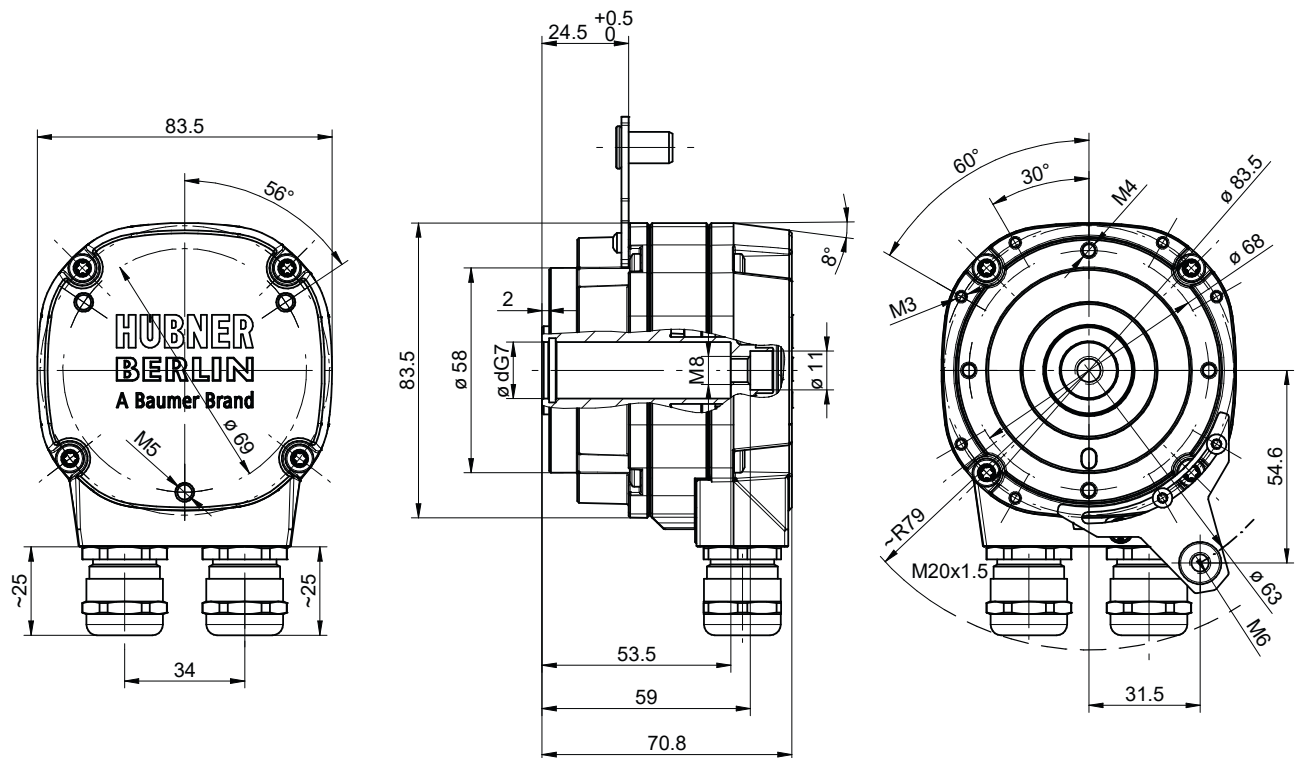
Abb. 18: Abmessungen der einseitig offenen Hohlwelle (Abmessungen in mm, wenn nicht anders angegeben)
