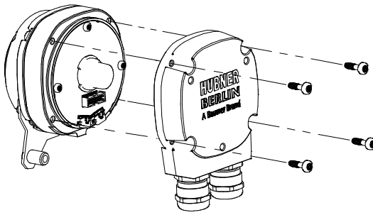
Abb. 4: Klemmenkasten demontieren
