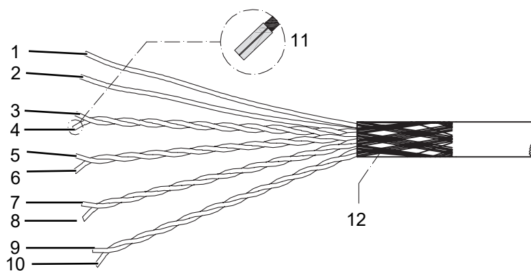
Abb. 9: Sensorkabel HEK 8
