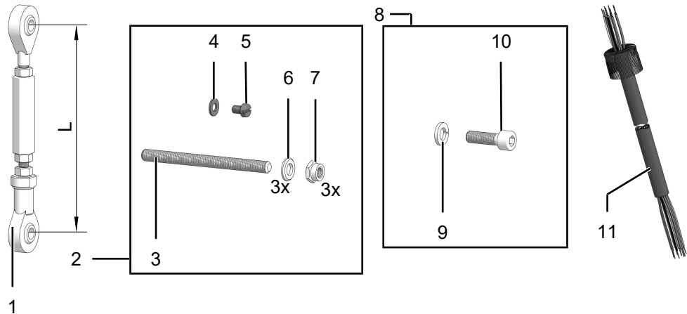
Abb. 1: Montagezubehör
