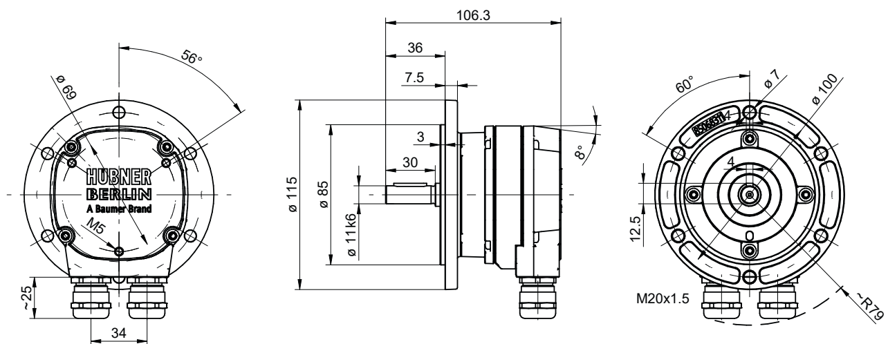
Abb. 19: Abmessungen der Vollwelle (Abmessungen in mm, wenn nicht anders angegeben)
