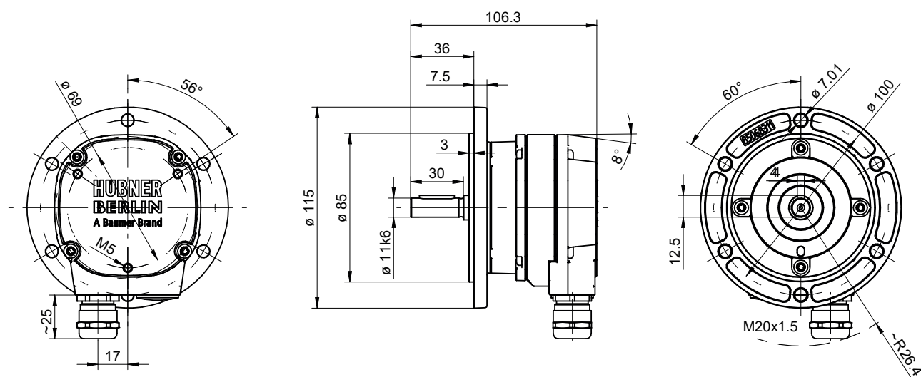
Abb. 17: Abmessungen der Vollwelle (Abmessungen in mm, wenn nicht anders angegeben)
