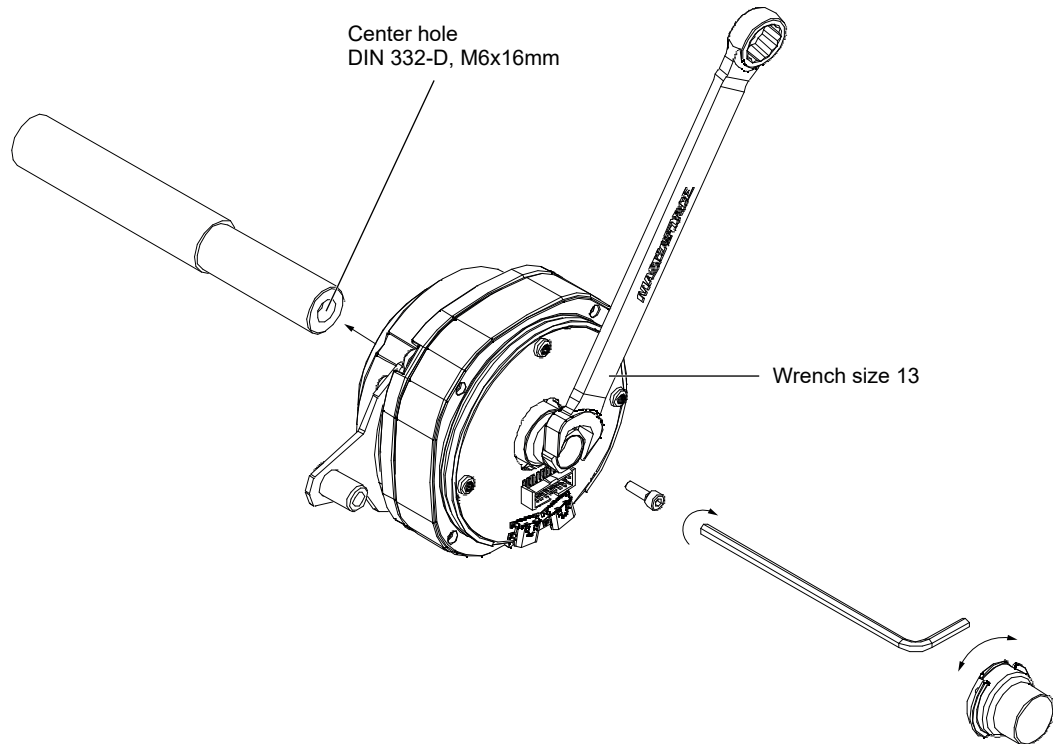
Abb. 5: Drehgeber montieren
