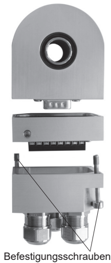
Befestigungsschrauben
